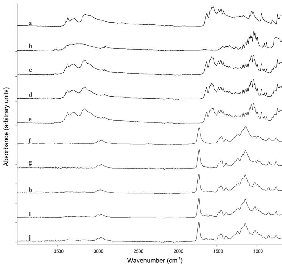
Fig. 1. FTIR spectra of: (a) metformin hydrochloride, (b) \alpha -lactose monohydrate, (c) F1 IR, (d) F2 IR, (e) F3 IR, (f) Eudragit® RL100, (g) Eudragit® RS100, (h) F1 PR, (i) F2 PR, and (j) F3 PR
