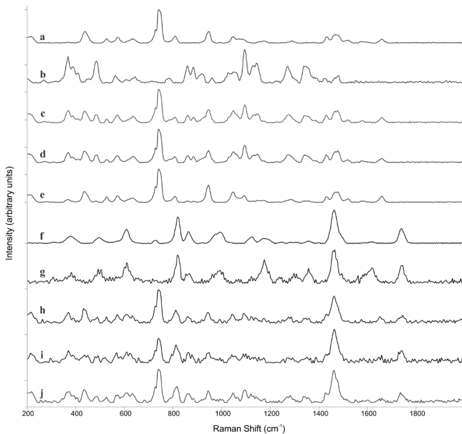
Fig. 2. Raman spectra of: (a) metformin hydrochloride, (b) \alpha -lactose monohydrate, (c) F1 IR, (d) F2 IR, (e) F3 IR, (f) Eudragit® RL100, (g) Eudragit® RS100, (h) F1 PR, (i) F2 PR, and (j) F3 PR
